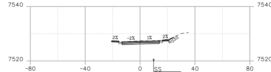
STA. 59+20
