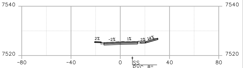
STA. 59+61
