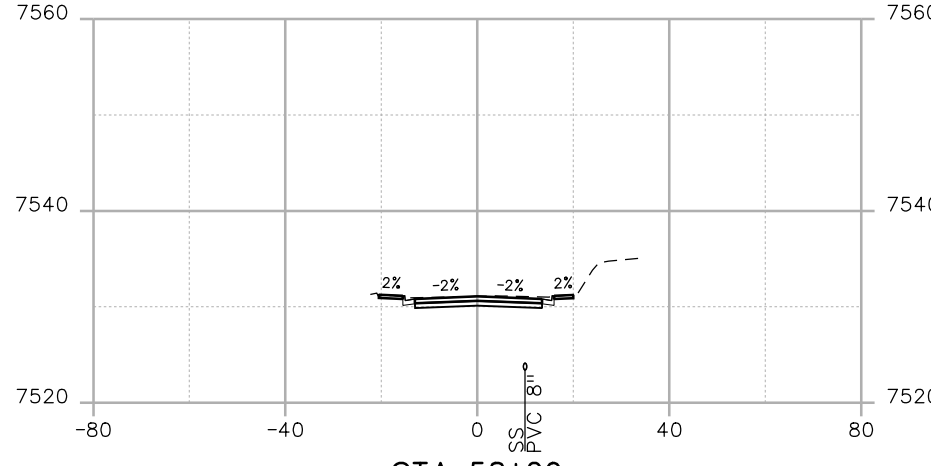
STA. 58+20
