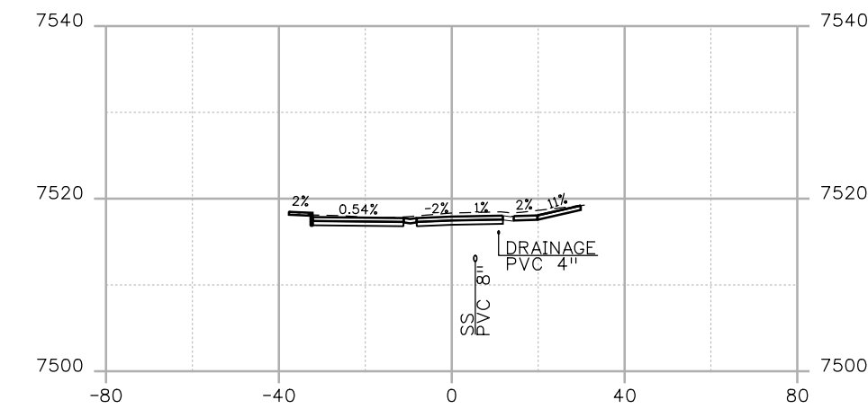
STA. 61+35
