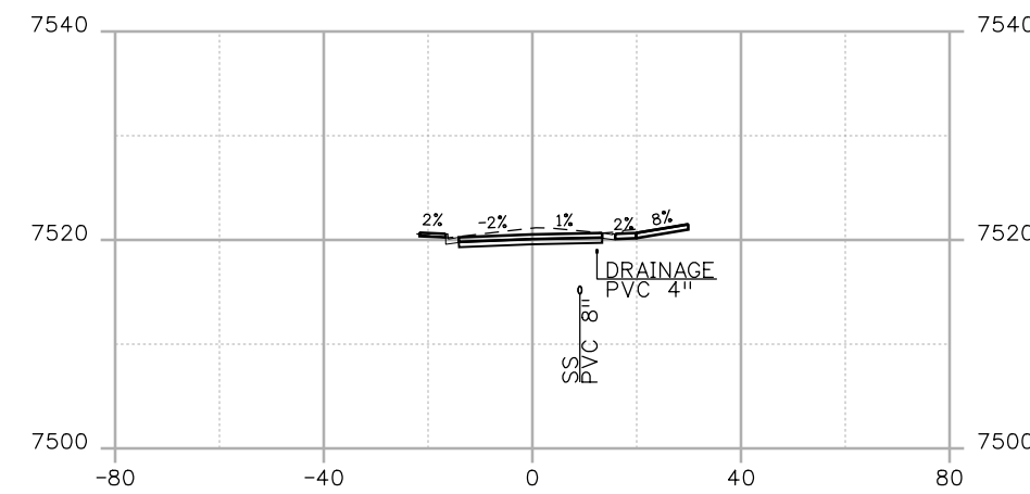
STA. 60+75
