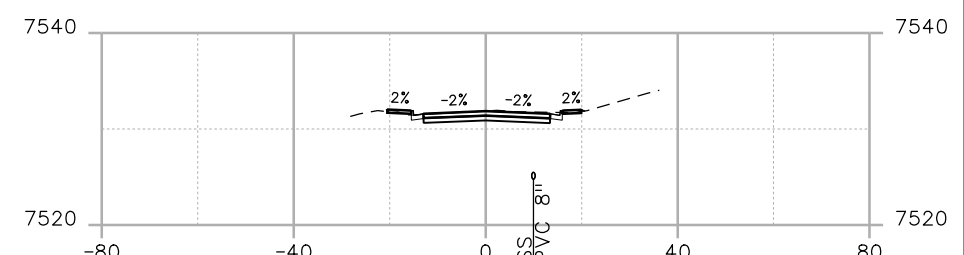
STA. 57+80
