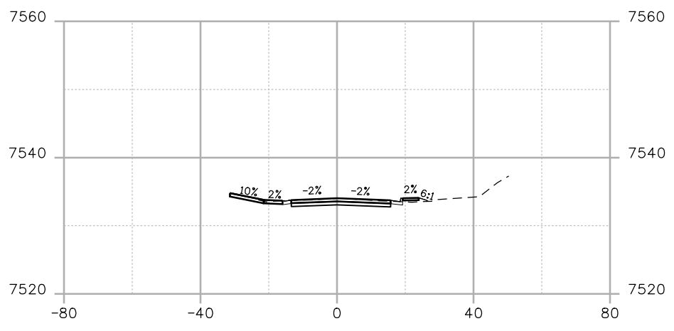
STA. 55+97
