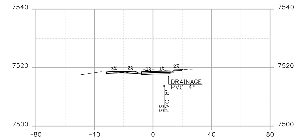
STA. 61+17
