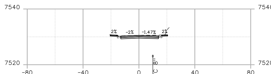
STA. 58+40
