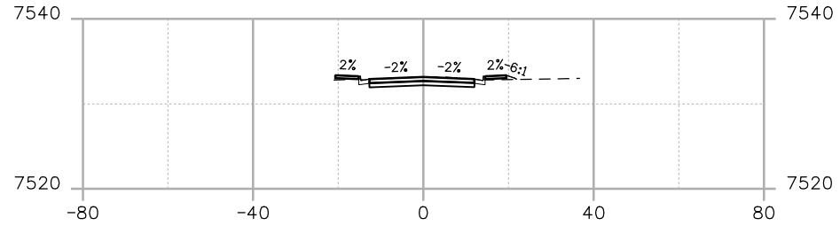
STA. 56+60
