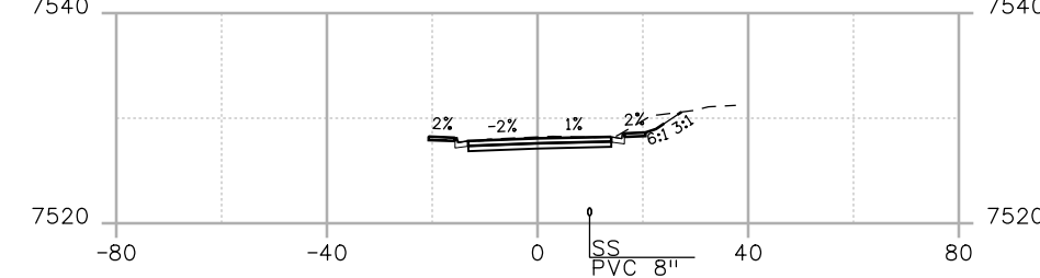
STA. 59+00
