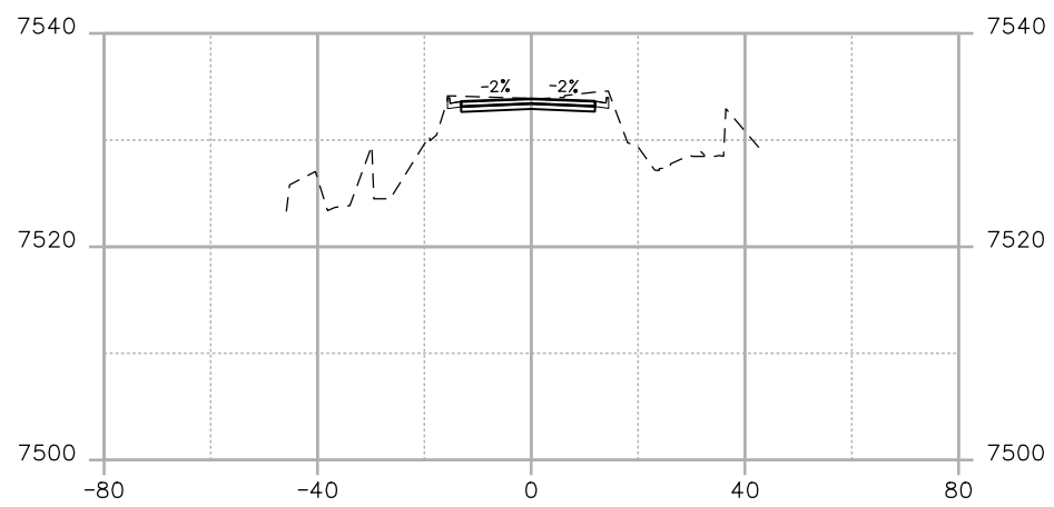
STA. 56+20
