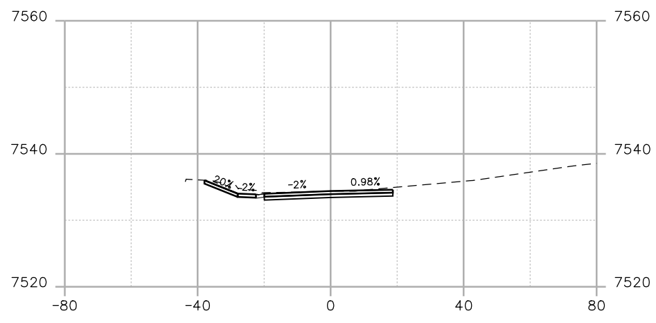
STA. 54+22
