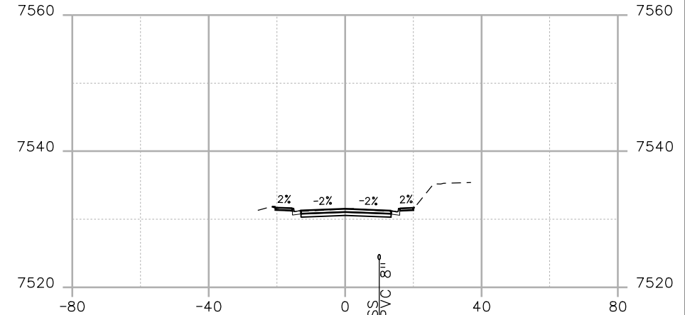
STA. 58+00
