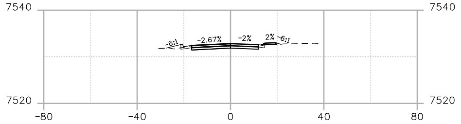
STA. 56+80
