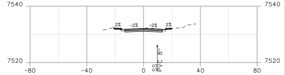
STA. 57+60
