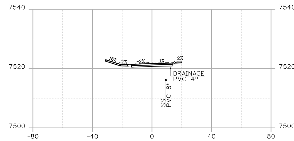
STA. 60+48
