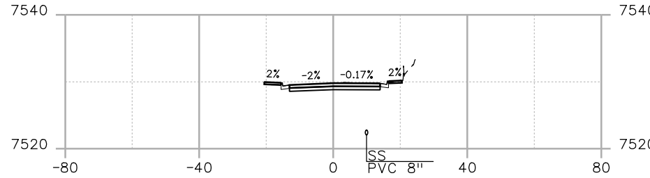
STA. 58+60
