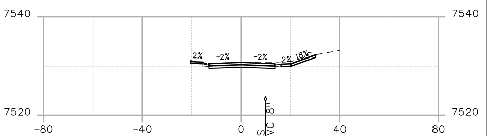
STA. 58+32
